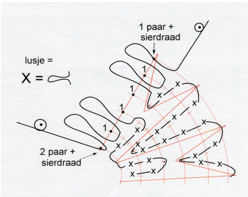
Werktekening hart met lussen
